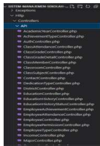
Gambar 5 Struktur kode
