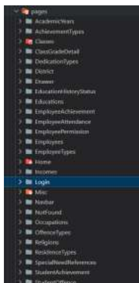
Gambar 3.1. Struktur Kode
