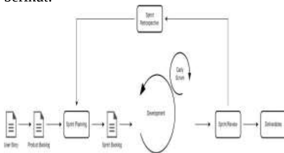
Gambar 2 Perancangan Luaran dengan Framework Scrum (2022)
